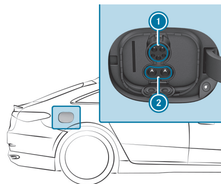
Fahrzeugsteckdose Typ Combo 1
