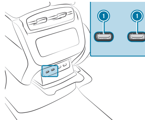
USB-Anschlüsse im Elektronikfach in der Mittelkonsole im Fond (Beispiel)
