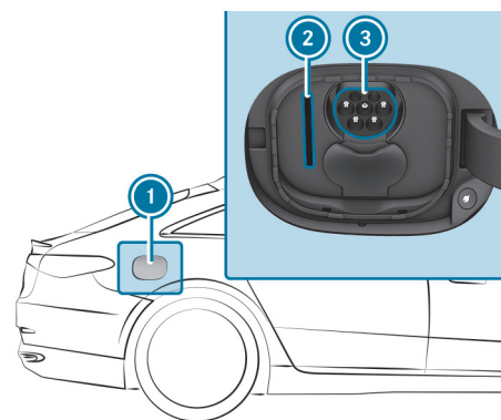
Fahrzeugsteckdose Combo 2
