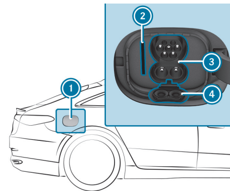
Fahrzeugsteckdose Combo 2
