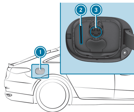
Fahrzeugsteckdose Combo 1
